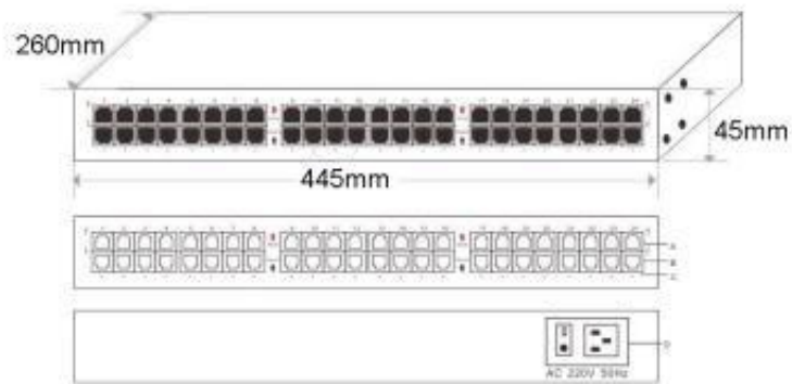
A. RJ45 PoE 输出口 B. RJ45 输入电口 C. PoE 指示灯 D. AC 220V/50Hz
