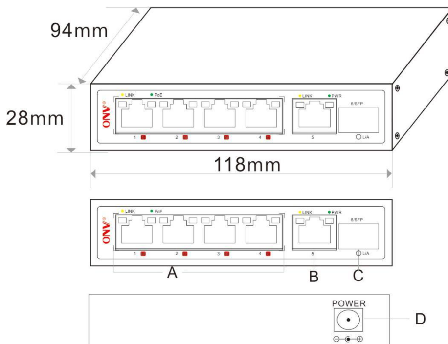
A. 4个bt PoE供电口 B. 上联电口 C. 上联光口 D. Dc电源接口
